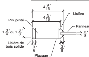
BATTANT PANNEAU PLAT #29XX
