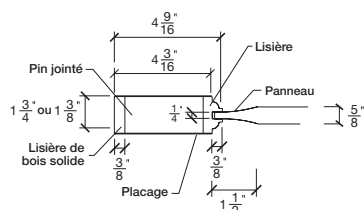
BATTANT PANNEAU PROFILÉ #20XX
