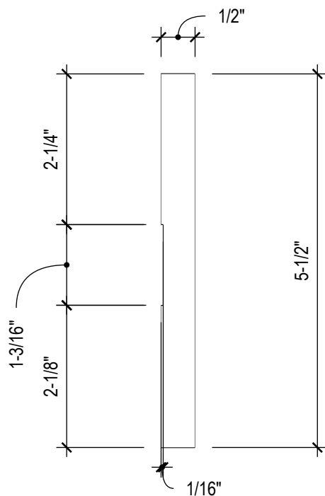
3 COUPE 1 Échelle: 1:1
